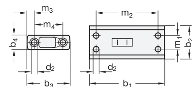
Rozměry pro instalaci (pohled shora)
