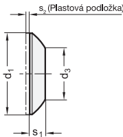
Plastová podložka
