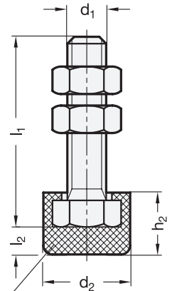
Ochranná krytka GN 806
