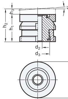
Zátěžová podložka GN 6339
