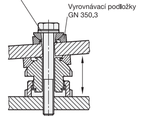
Zátěžová podložka GN 6339
